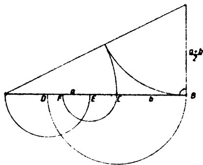
Abbildung 1.11. Geometrische Konstruktion des Goldenen Schnitts
