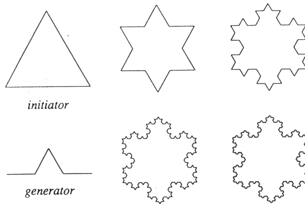
Abbildung 1.22. Schneeflockenkurve nach Koch
