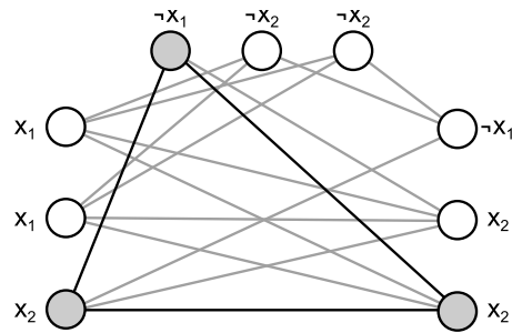
Abbildung 8.4: Beispiel: Reduktion einer 3-KNF Formel mit 3 Klauseln auf einen Graph mit einer 3-Clique
