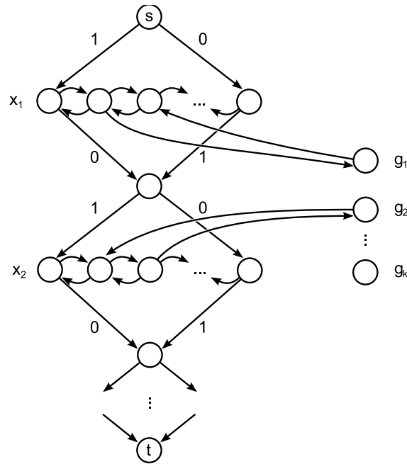
Abbildung 8.5: Veranschaulichung der Reduktion von 3SAT auf HAMILTON
