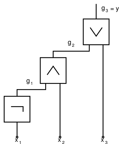
Abbildung 7.2: Beispiel eines booleschen Schaltkreises
