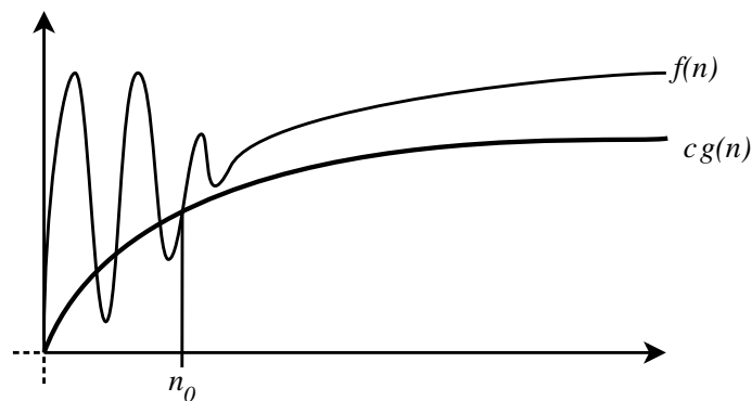
Abbildung 0.4: Asymptotisch obere Schranke
