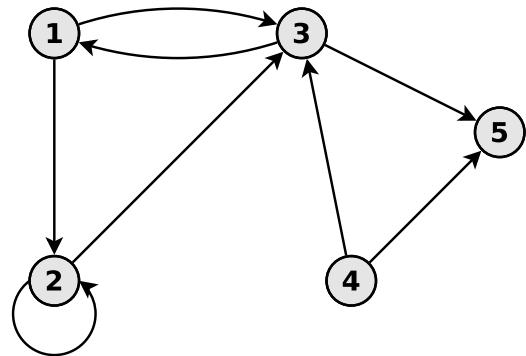
Abbildung 0.15: Graph G'
