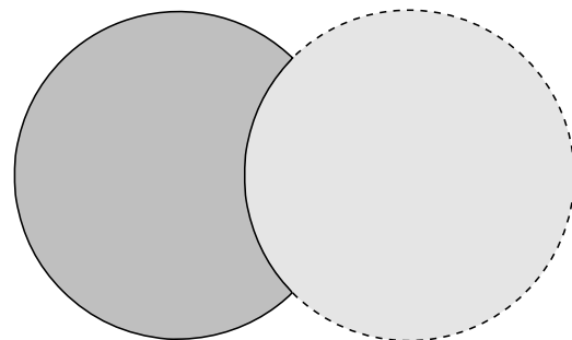
Abbildung 0.3: Differenzmenge
