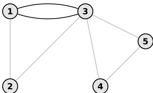
Abbildung 0.10: Mehrfachkante
