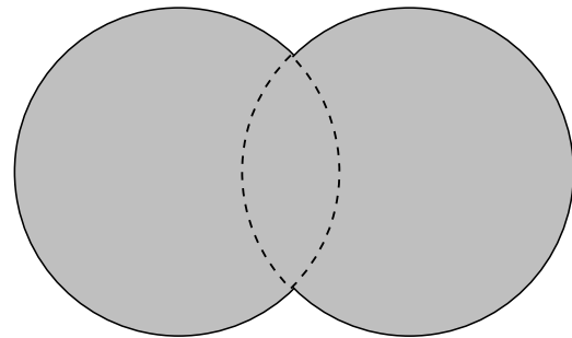
Abbildung 0.2: Vereinigungsmenge
