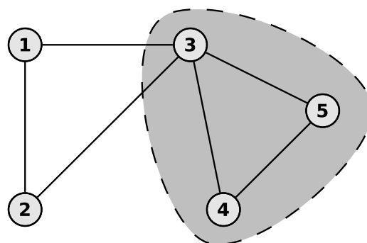
Abbildung 0.12: Clique der Größe 3
