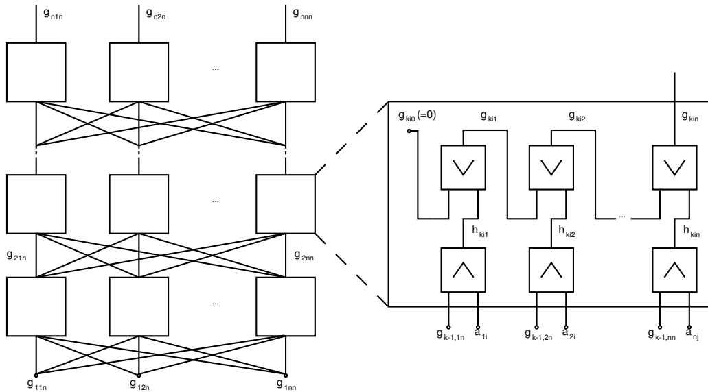
Abbildung 7.3: Beispiel Reach-Circuit Graph
