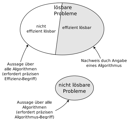
Abbildung 1.1: Intuitive Berechenbarkeit
