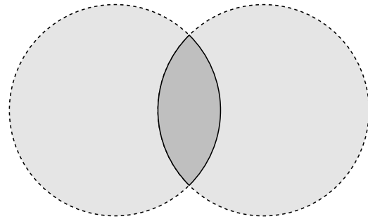
Abbildung 0.1: Schnittmenge
