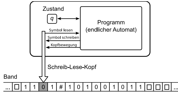
Abbildung 3.1: Schematische Darstellung einer Turingmaschine
