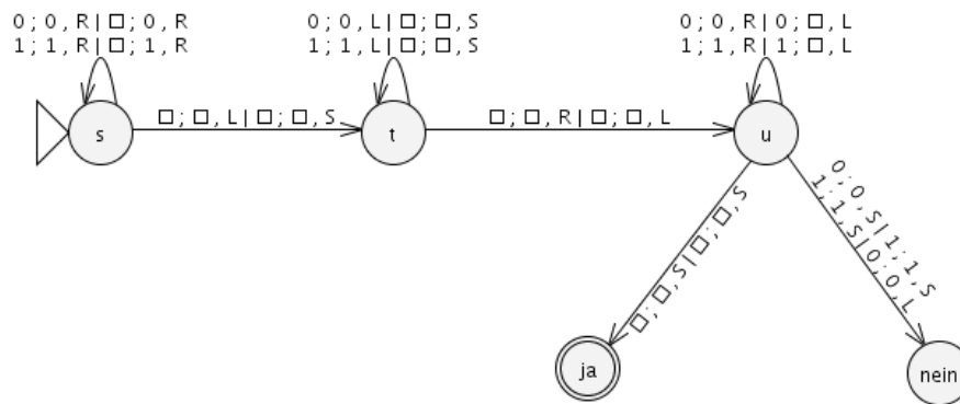
Abbildung 3.2: Turingmaschine für Palindrom-Entscheider
