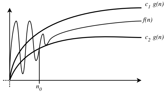
Abbildung 0.6: Asymptotisch exakte Schranke
